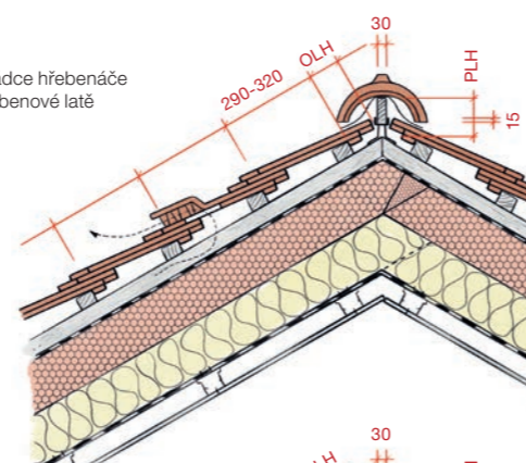
Korunové krytí
