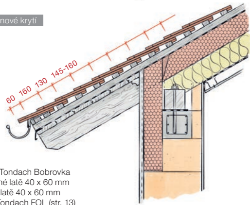
LAŤOVÁNÍ V ZÁVISLOSTI NA SKLONU STŘECHY
