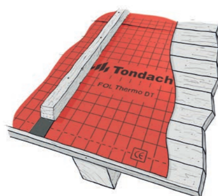
třída těsnosti 3
