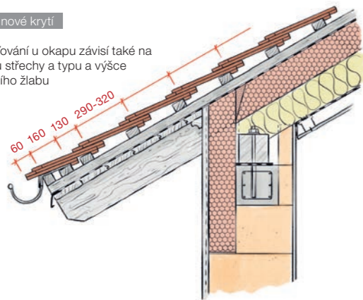
Šupinové krytí
