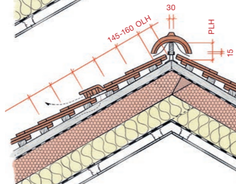
Šupinové krytí
