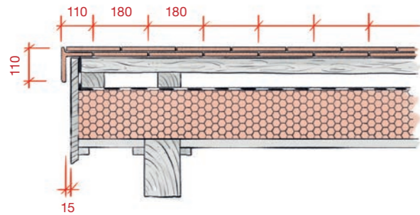
OKAP
